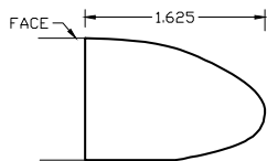
Alpha Edge | WE06
