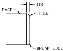
Wood Edge | WE01 Standard
