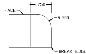
Waterfall Edge | WE03
