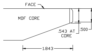
Knife Edge | WE07
